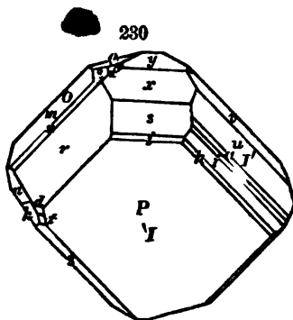
Axinite.
